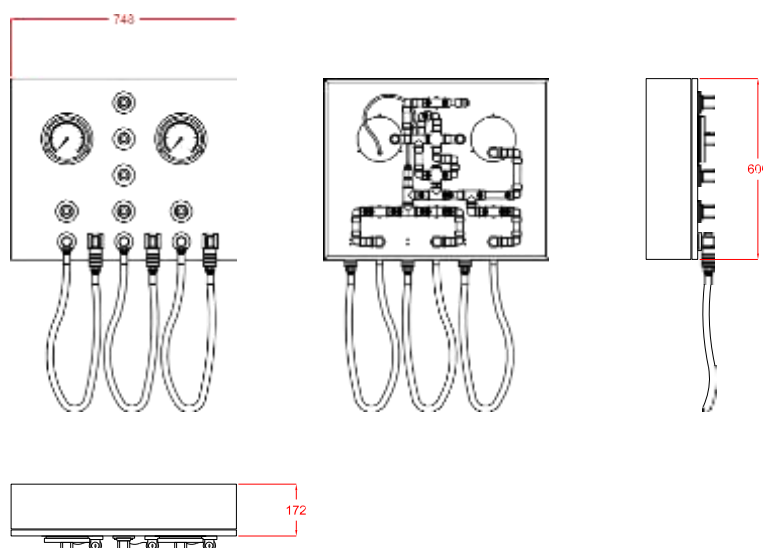
Dibujos técnicos* - Technical illustrations* - Données techniques*
