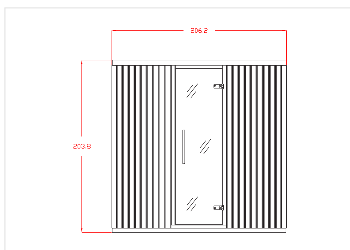
Alzado - front - Plan en élévation
